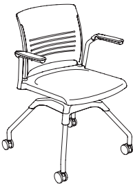
L2SNPCANAR
