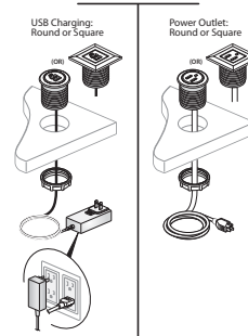
Bezel Utility Module EURT-0072-1100 EURT-0072-1010
