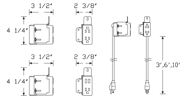
Grommet Mount
